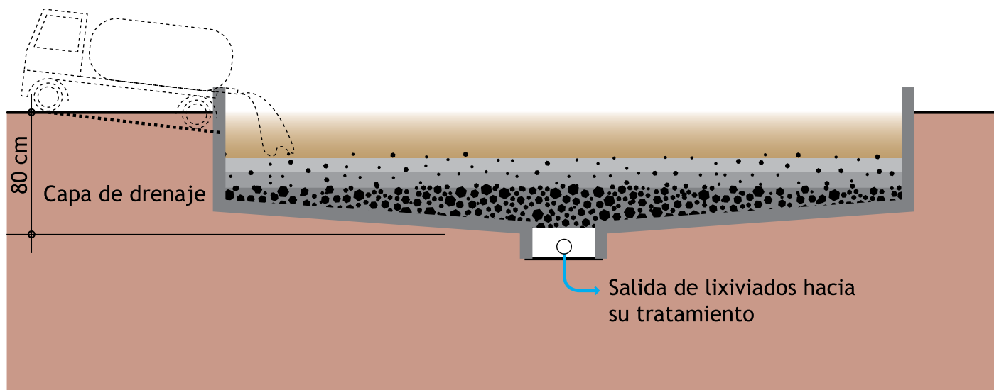
Figura 7.1 Esquema de un lecho de secado sin plantas (Tilley et al., 2014). Si bien no se le observa en esta figura, un deflector es esencial para dispersar la fuerza del chorro de lodos y proteger la arena (Sección 7.5).
