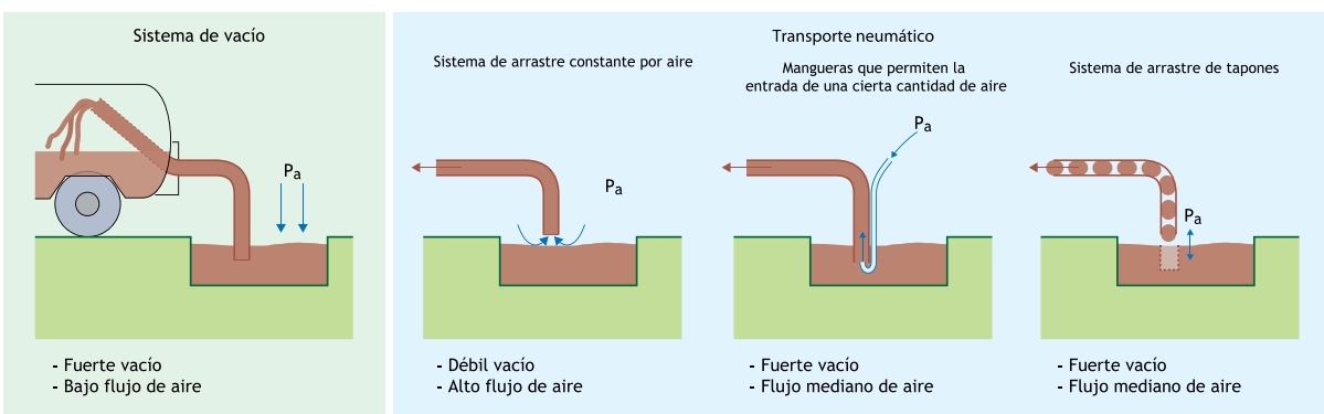
Figura 4.9 Cuatro tipos de técnicas para aspirar los lodos (adaptado de Böesch y Schertenleib, 1985)
