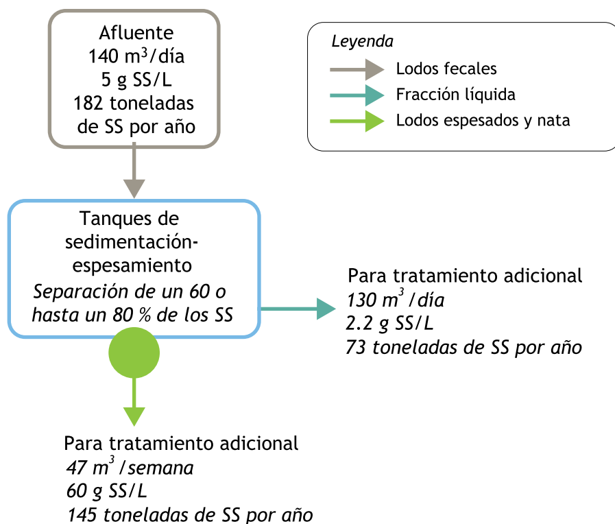
Figura 6.9 Esquema de los flujos de masa en el ejemplo teórico de tratamiento en tanques de sedimentación-espesamiento.
