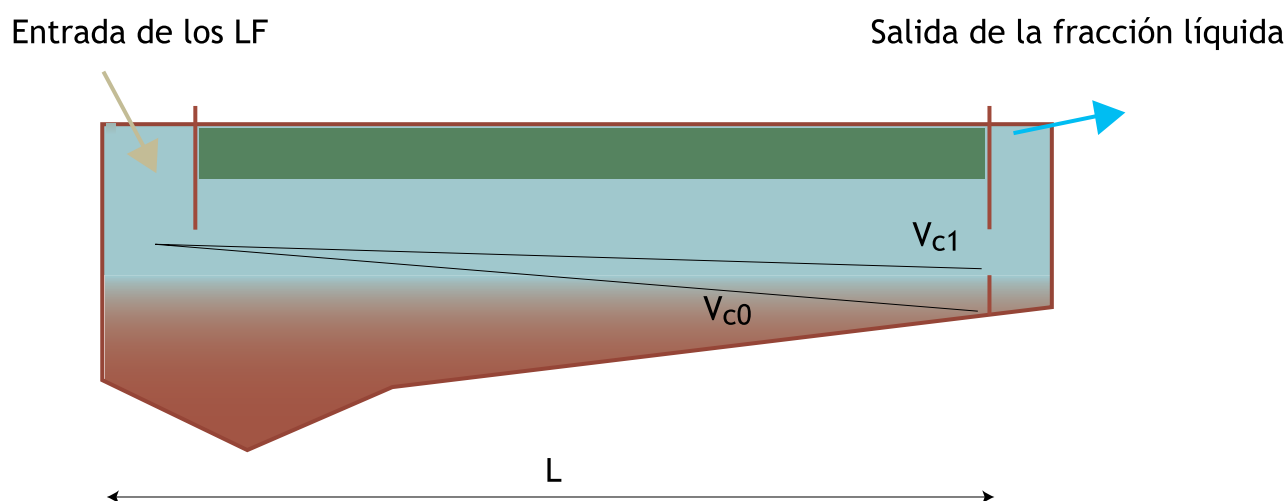
Figura 6.3 Esquema de la velocidad final de sedimentarse ( V_c ) requerida para que una partícula se asiente dentro de un tanque de longitud L .
