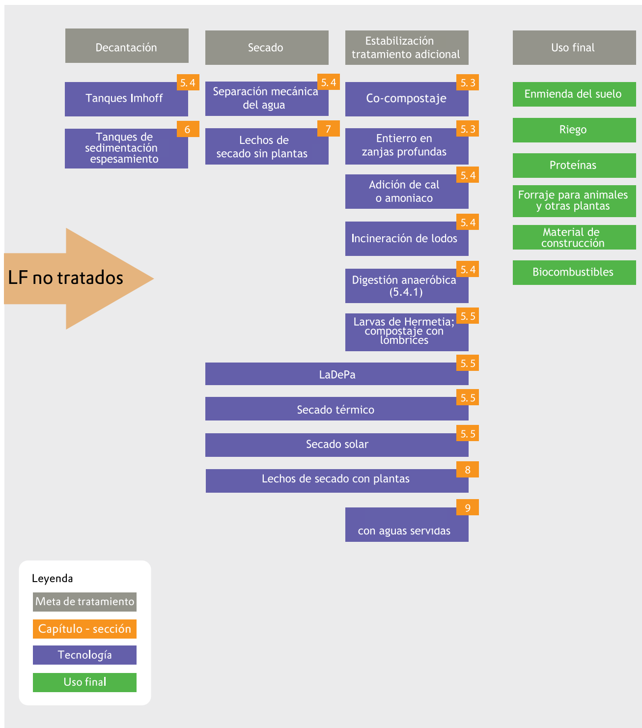
Figura 5.1 Categorización de las tecnologías de tratamiento según sus metas de tratamiento. Los productos finales son analizados en el capítulo 10. Los flujos específicos de una tecnología a otra se presentan en el esquema para la selección de tecnologías en la figura 17.10.
