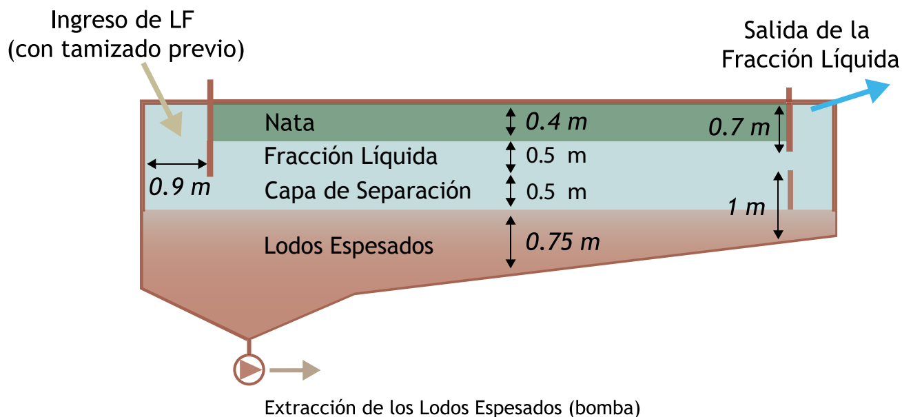
Figura 6.8 Esquema de la configuración del tanque de sedimentación-espesamiento del ejemplo de diseño.
