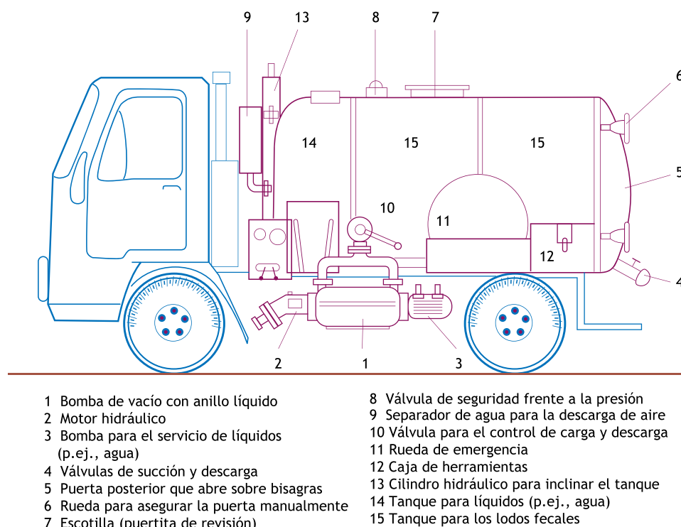
Figura 4.10 Esquema del camión aspirador BREVAC (adaptado de Böesch y Schertenleib, 1985)
